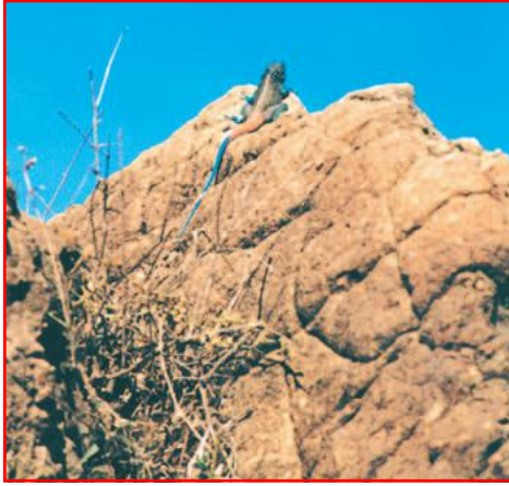
شكل ( ٤٠ ) تجوية ميكانيكية
