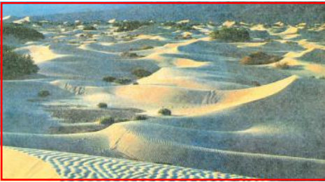
شكل (٤٣) أثر التعرية بالرمال
